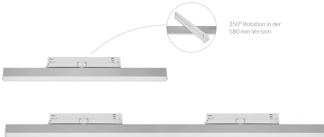
Standardmodell: Profil Aluminium eloxiert, Adapter weiss
